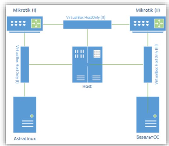
Рисунок 1 – Конфигурация сети для практического занятия
